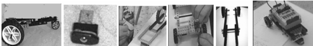
Εικόνα 13: Πορεία κατασκευής τρικύκλου
