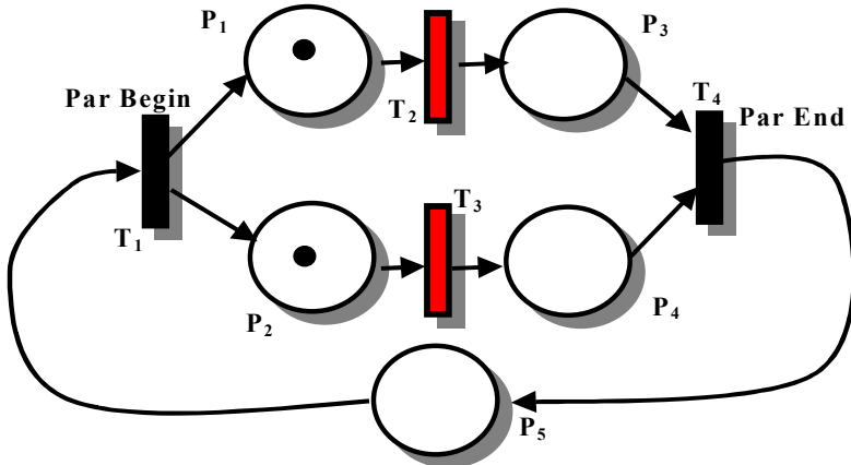
Σχήμα 3. Παράλληλια και συγχρονισμός στα δίκτυα Petri
