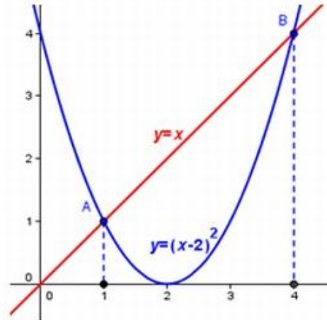
Γραφική λύση της x = (x - 2)^2
