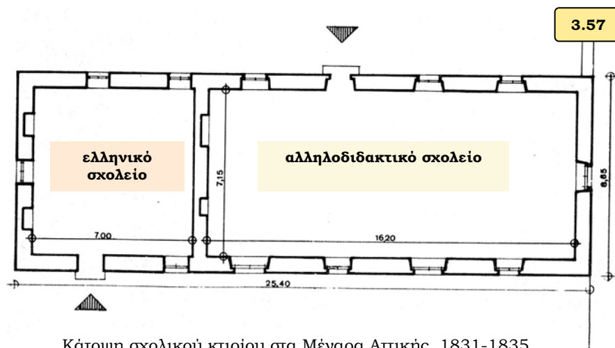
Κάτοψη σχολικού κτιρίου στα Μέγαρα Αττικής, 1831-1835
