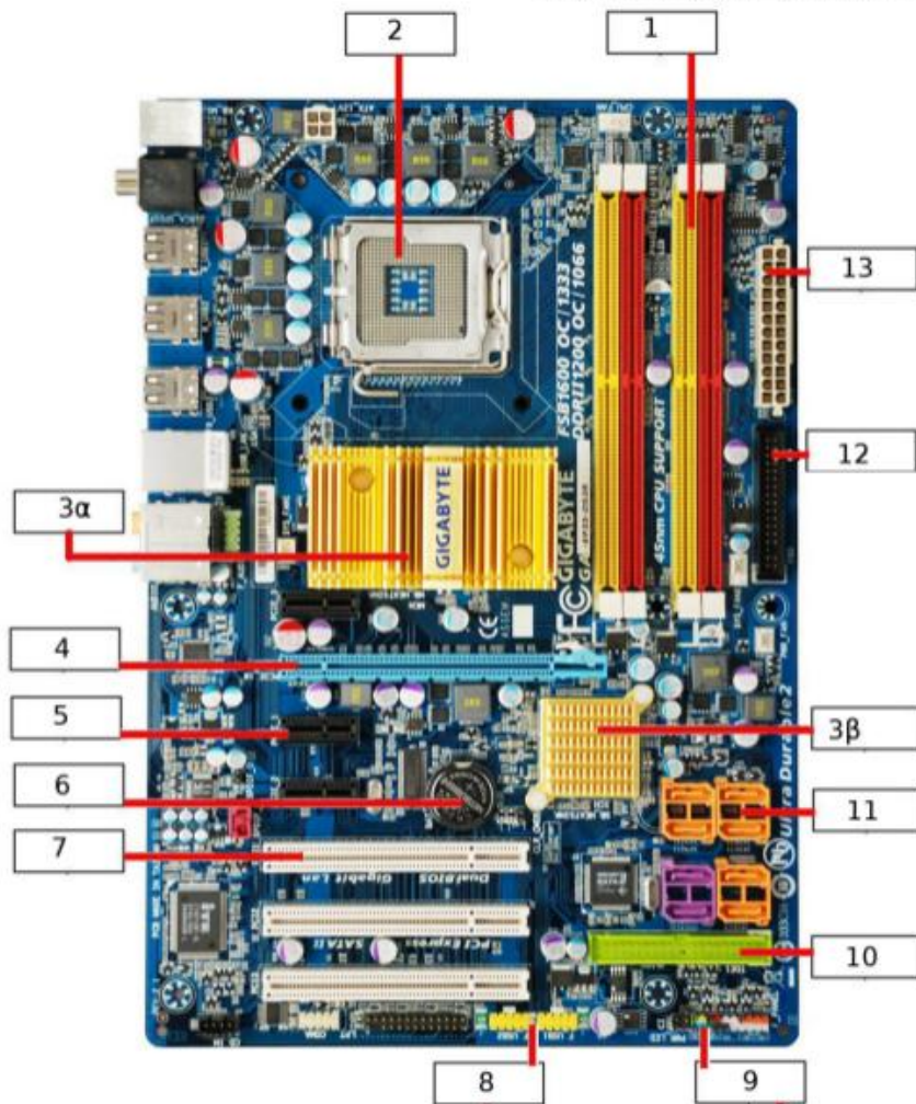
Εικόνα Α - Κάτοψη Μητρικής
